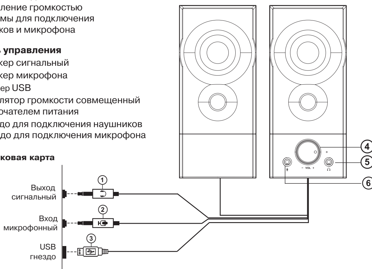
Рис. 1. Схема подключения
